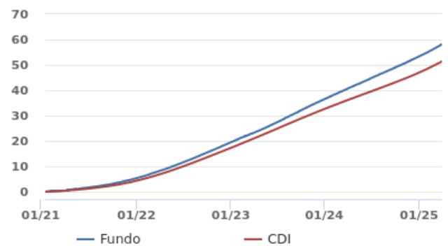
Retorno Acumulado (% Efetivo)
