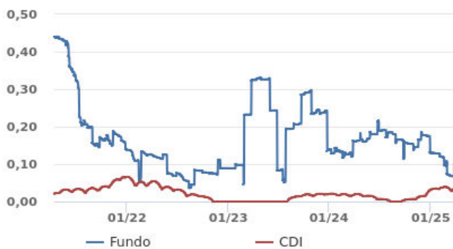
Volatilidade Anualizada (%): Janelas Móveis de 63 du
